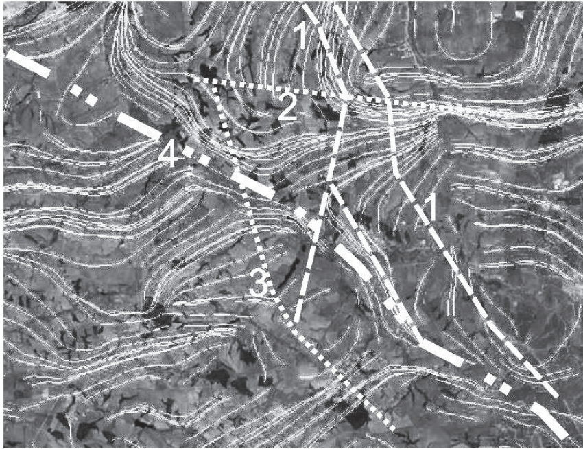
Рис. 4. Выраженность основных зон разломов: Железногорского (1), Субширотного (2) и Безымянного (3), а также мезозойской флексуры (4) в линеamentных формах
