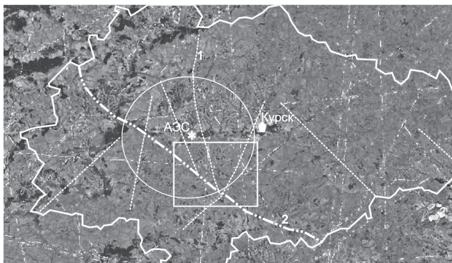
Рис 2. Линеamentный анализ территории Курской области. Белая врезка – район детальных исследований, окружность – 30 км зона. Показаны, выделенные LESSA, протяжённые линеamentы; вынесены активные верхнемеловые разломы (белые прерывистые линии). 1 – Железнодорожный разлом, 2 – верхнемеловая флексура
