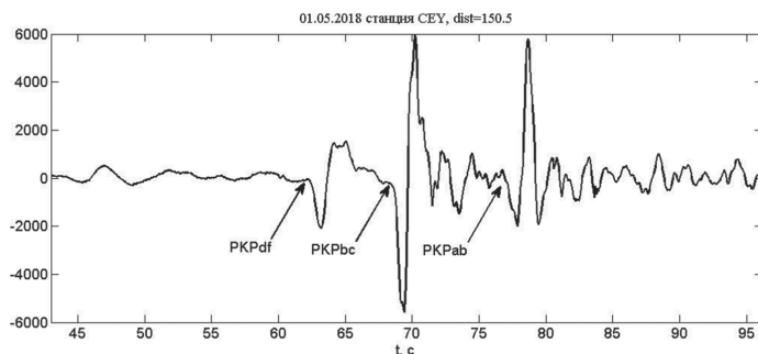
Рис. 1. Фрагмент сейсмограммы землетрясения на овах Фиджи 01.05.2018 г., зарегистрированной сейсмической станцией CEY на эпицентральной расстоянии 150.5^\circ
